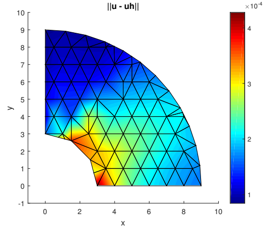
(d) Pressurized cylinder - FEM
